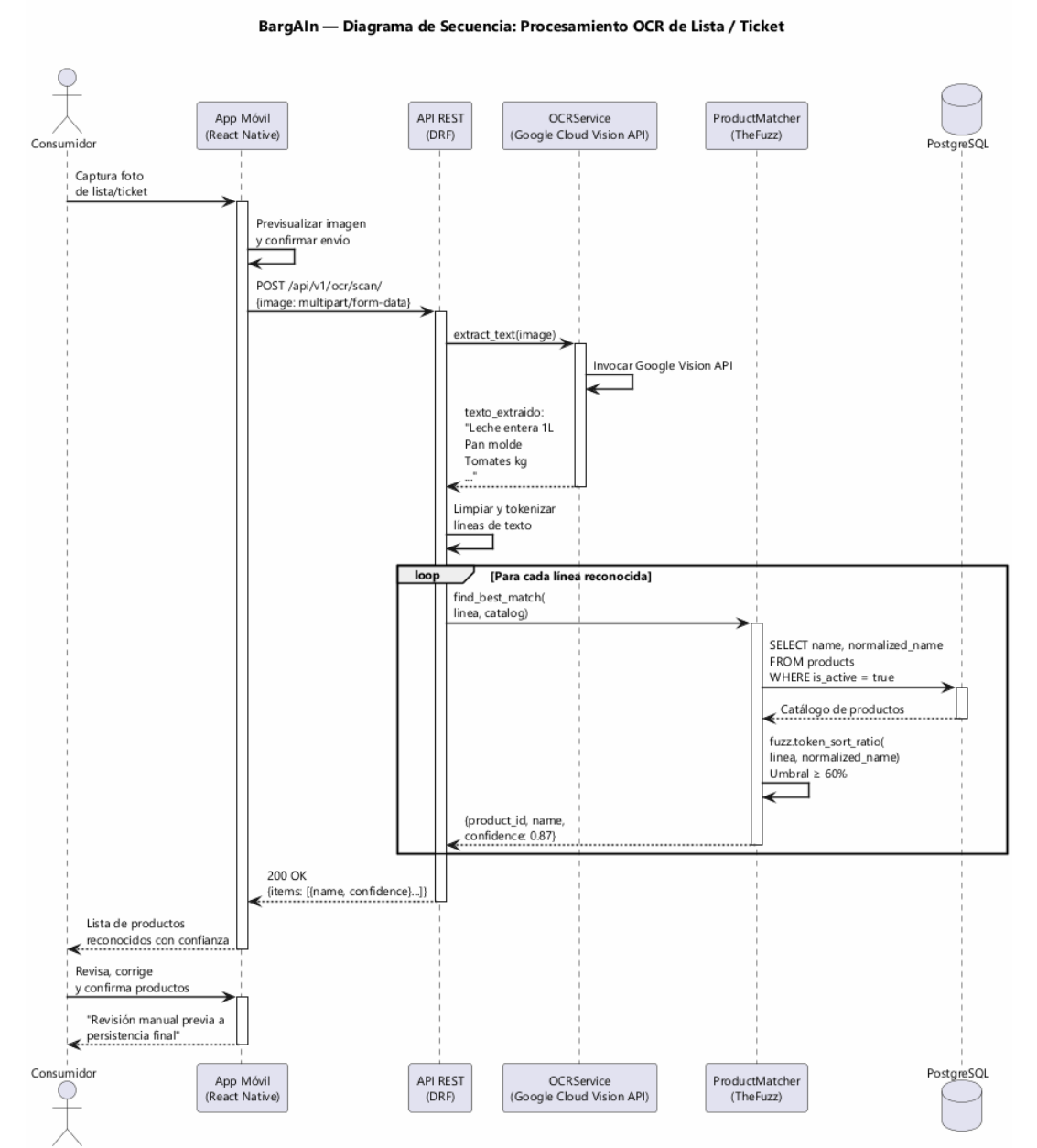
Figura 6.5: Diagrama de secuencia del flujo OCR
